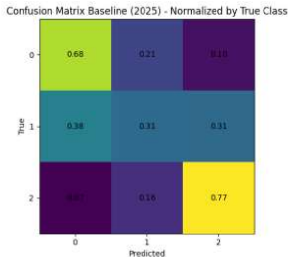
Gambar 4. Confusion matrix model baseline pada data uji 2025
