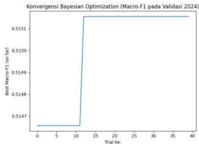
Gambar 5. Kurva konvergensi Bayesian Optimization (Optuna) berdasarkan macro-F1 pada data validasi 2024
