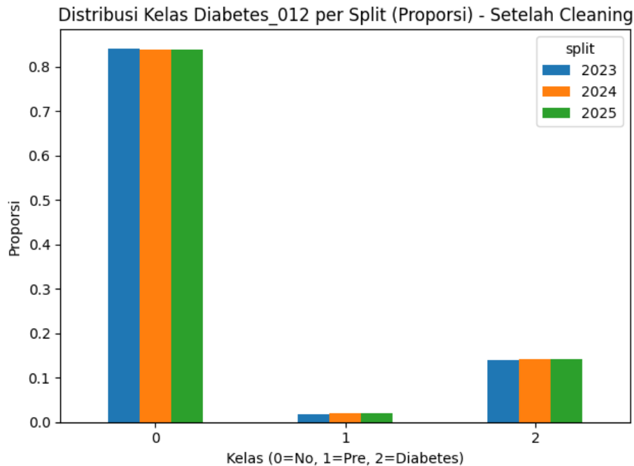
Gambar 6. Distribusi kelas Diabetes_012 pada masing-masing subset setelah preprocessing.
