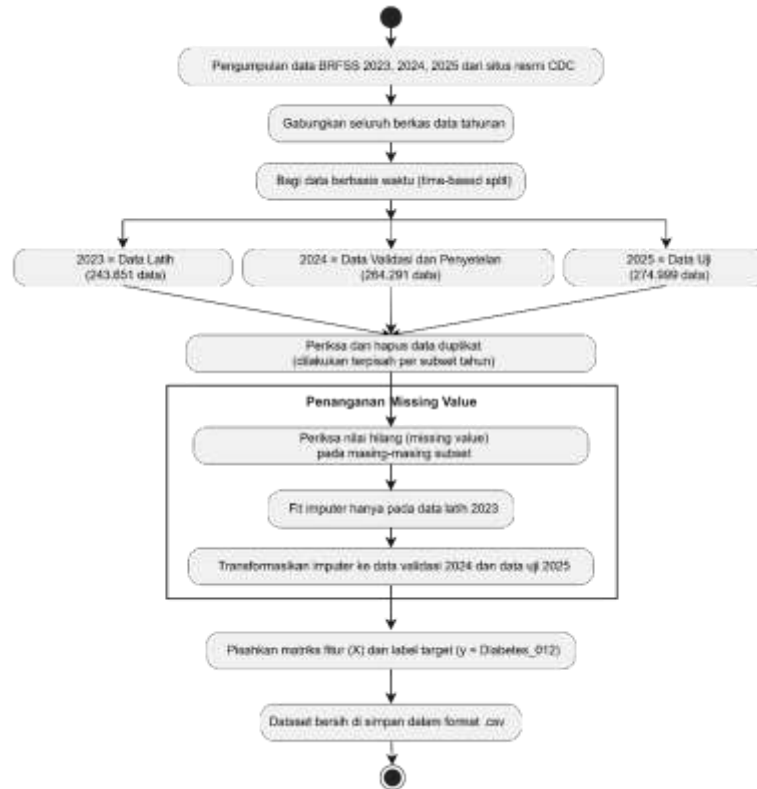
Gambar 2. Diagram alur tahapan pengumpulan dan preprocessing data
