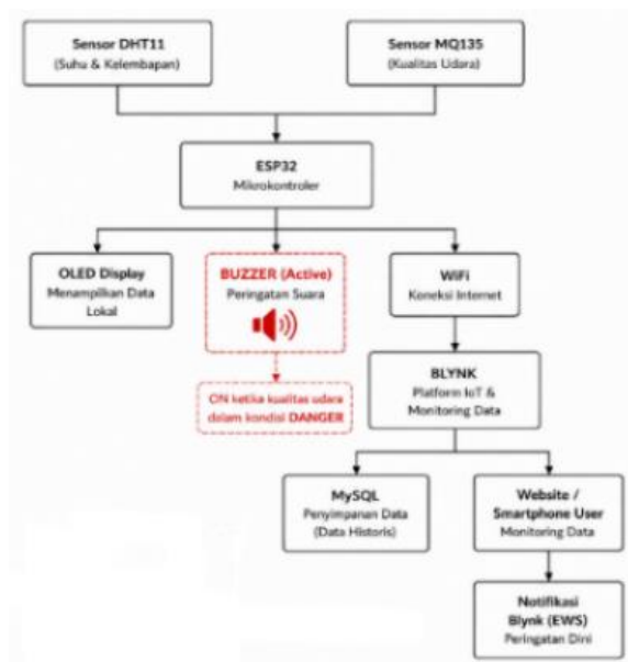
Gambar 4. Diagram Blok Sistem Monitoring Kualitas Udara
